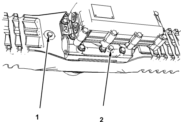
Рисунок 2 Задний дифференциал (1) Пробка контрольно-наливного отверстия (2) Пробка сливного отверстия g01357819
