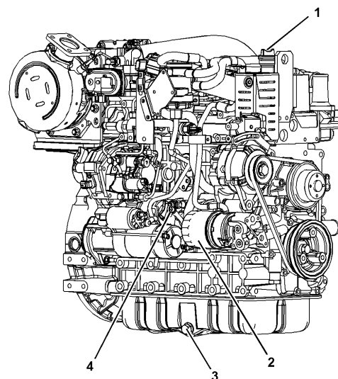
Рисунок 1 (1) Крышка маслоналивной горловины (2) Масляный фильтр (3) Клапан для слива масла (4) Масляный щуп g03730932
