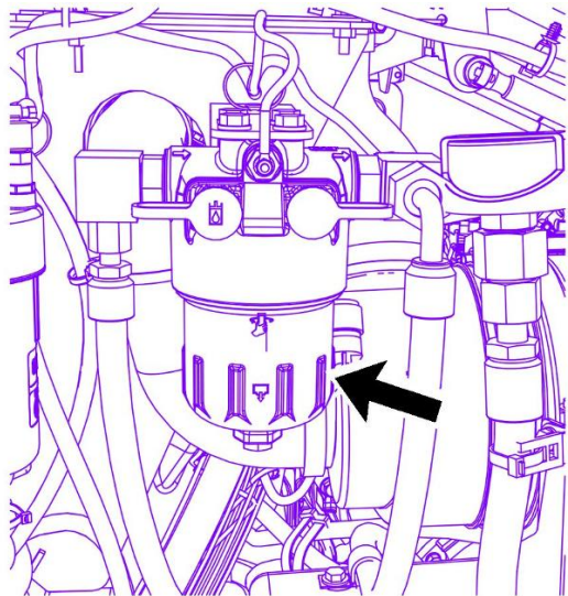
Рисунок 1 Масляный фильтр гидравлической системы g06293671
