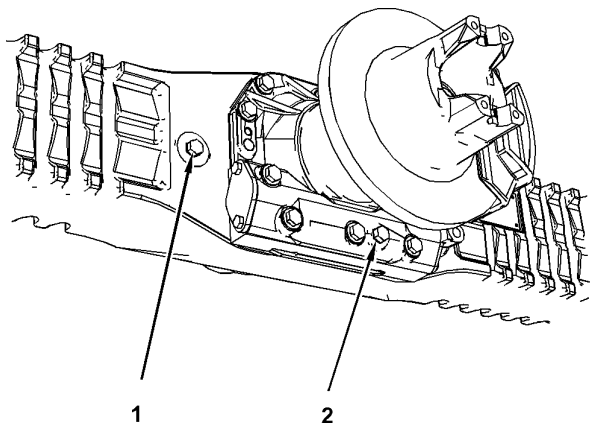
Рисунок 1 Передний дифференциал (1) Пробка контрольно-наливного отверстия (2) Пробка сливного отверстия g01357818
