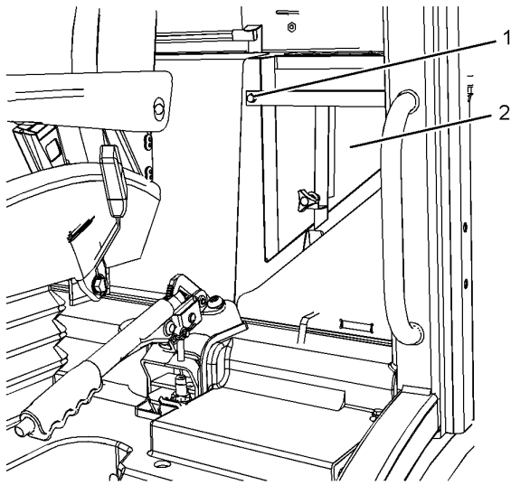
Рисунок 1 (1) Винты (2) Внутренний фильтрующий элемент g03805646
