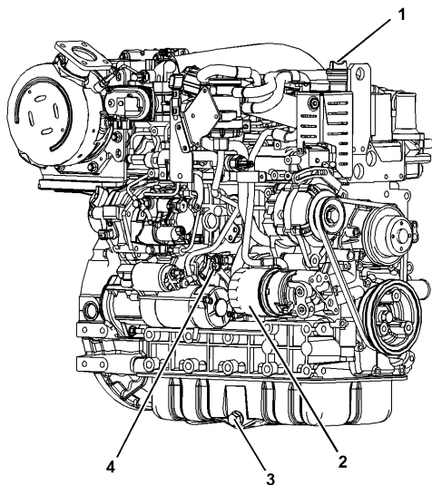
Рисунок 1 g03730932 (1) Крышка маслоналивной горловины (2) Масляный фильтр (3) Клапан для слива масла (4) Масляный щуп
